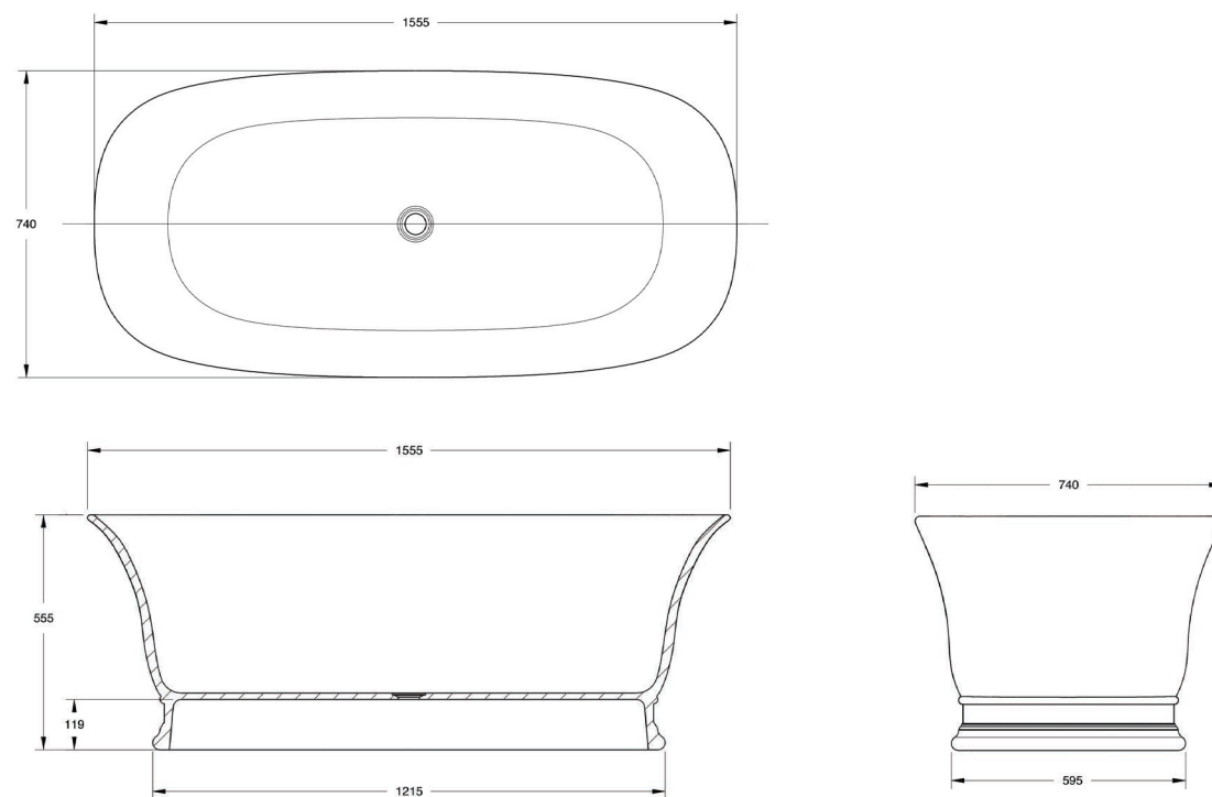
CAMBRIDGE 156 X 74 TITANCAST BATH
